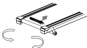
Vyrovnaní vychýlení pásu doprava ( diagram 3) Vyrovnaní vychýlení pásu doleva( diagram 4)
